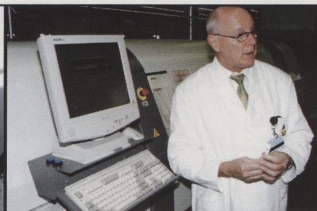
14 В этом довольно большом аппарате электронные элементы один за другим припаиваются к плате. Сложность в том, что нужна не только предельная точность, но и особая температура для каждого элемента.
