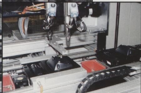
18 ...автоматические отвертки надежно свинчивают две половинки корпуса между собой.
