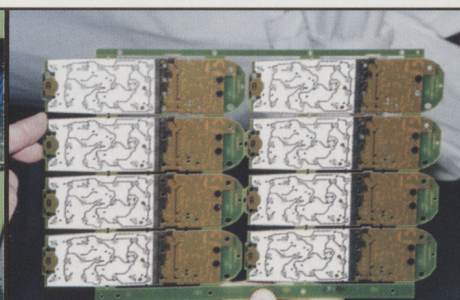
8 Параллельно на другой линии на печатные платы нанизывают всю необходимую электронику.
