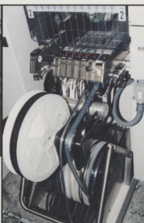
11 Большие электронные элементы также закреплены на перфоленте, скрученной в бобины.
