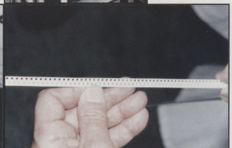
9 Отдельные элементы, которые требуется припаять к плате, размером меньше миллиметра. Они вставлены в специальную перфоленту, похожую на кинолентку. Установить их вручную невозможно.
