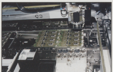
12 Станок-автомат наносит следующую порцию электронной начинки.
