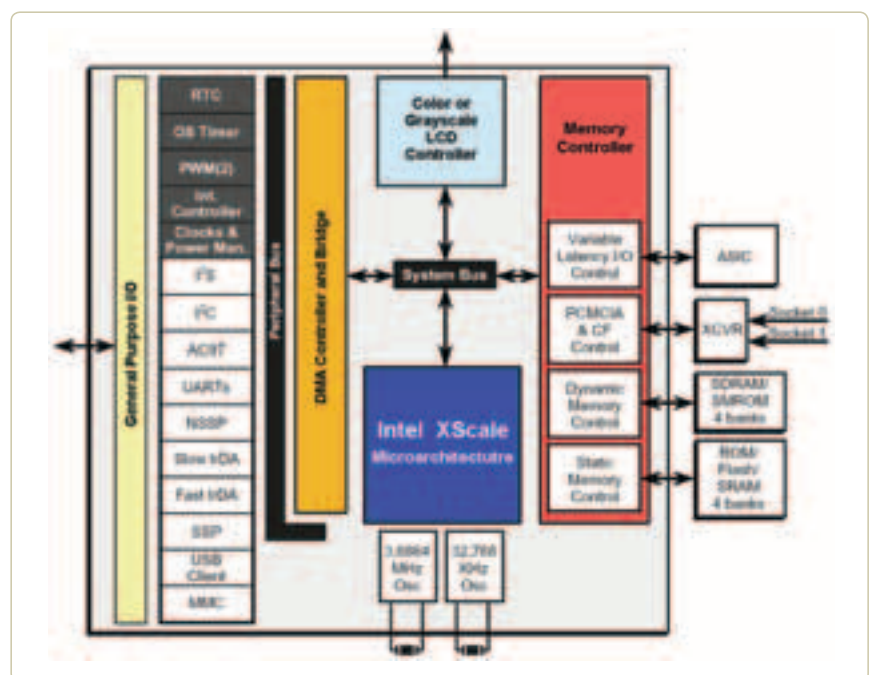
Функциональная схема процессора Intel PXA255
